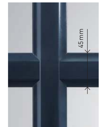
Cuarterones ALU - Disponibles en blanco, bicolor o monocolor Sección 45 x 8 mm
