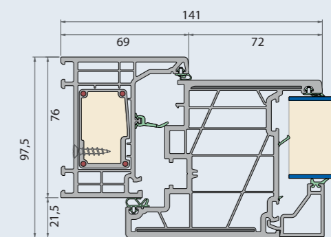
Sección horizontal
