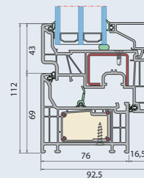
Sección vertical
