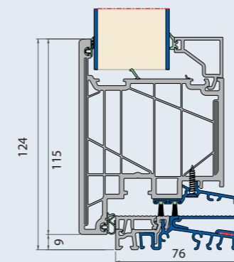
Sección vertical
