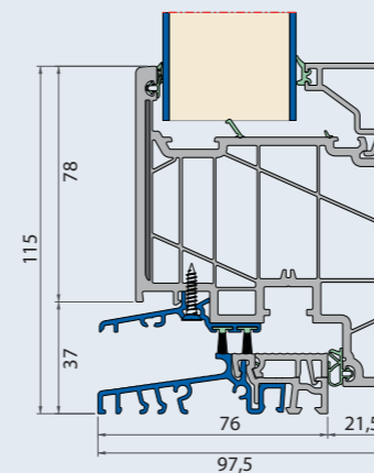
Sección vertical
